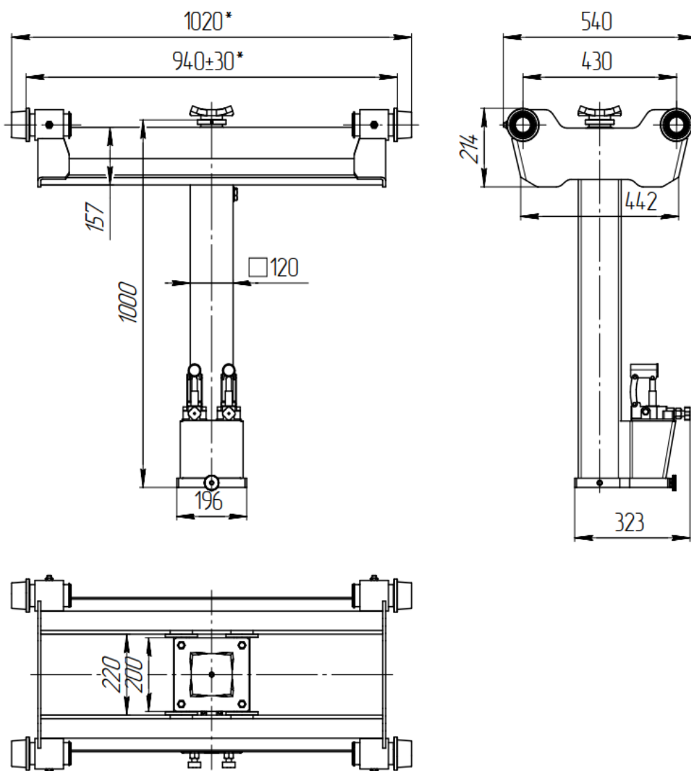
Рисунок 2 – Габаритные размеры и расстояние между опорными роликами
