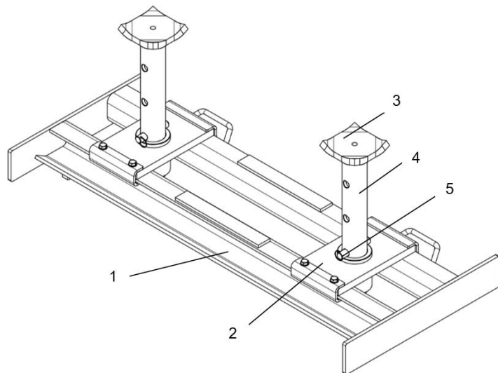
Рисунок 5 – Общий вид опорного моста 1 – рама; 2 – опорная плита; 3 – опора; 4 – удлинитель; 5 – фиксатор
