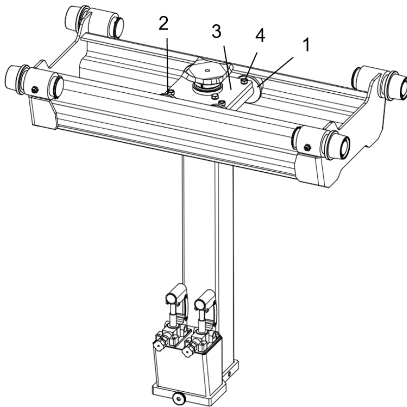
Рисунок 4 – Схема установки стойки на каретку
