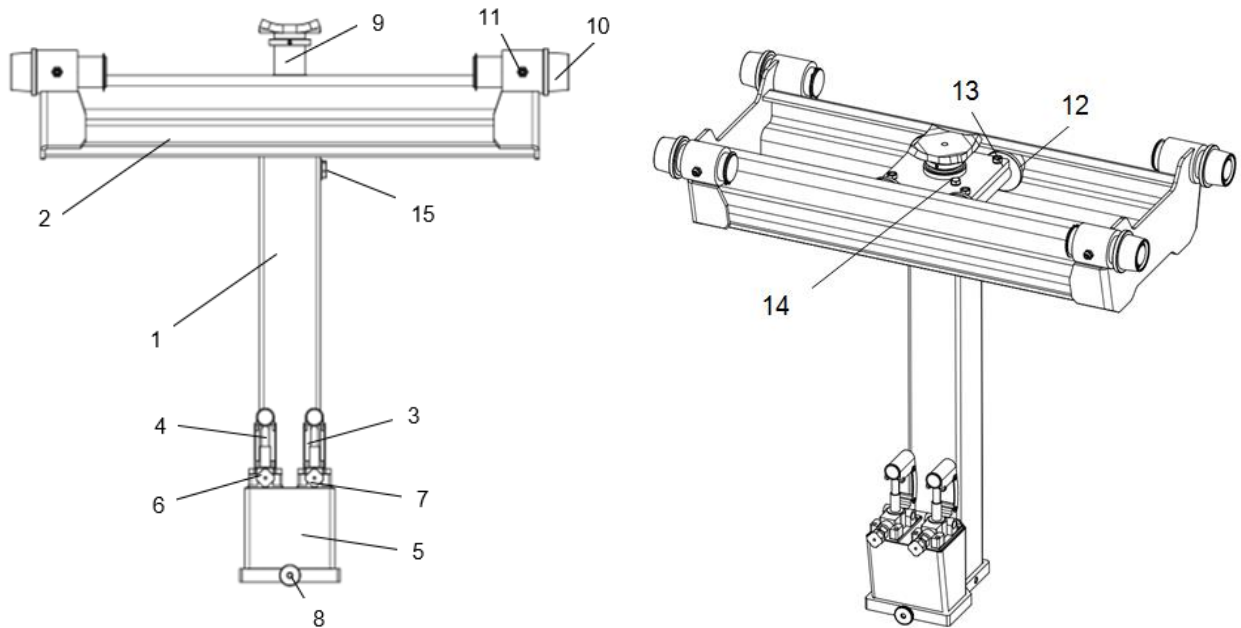
Рисунок 1 – Общий вид гидравлического домкрата
